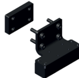
BLO-0466-48-01-00-0 Magneet blok (achterzijde) met verminderde kleeftkracht M6x25
