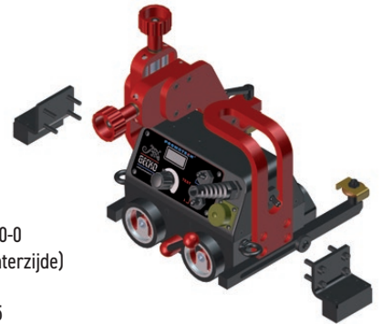
BLO-0466-47-01-00-0 Magneet blok (voorzijde) met verminderde kleeftkracht M5x25
