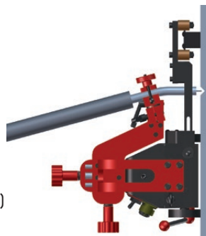
PRW-0466-50-02-00-1 Geleiderarmen voor flexibele rails (set van 2 stuks)
